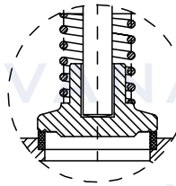
DN15....DN80
