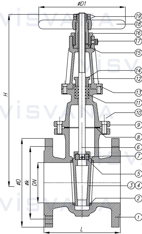
DN40...100 Wedge Type / Sürgü Tipi
