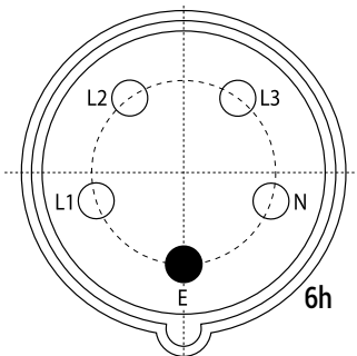
Prizin önden görünüşü Front view of receptacle
