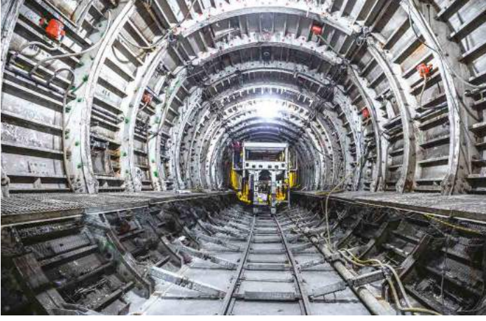
Tünel İnşaatı / Tunnel Construction
