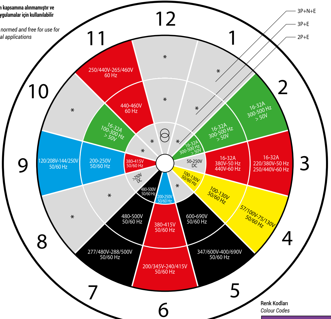
Prizin önden görünüşü Front view of receptacle
