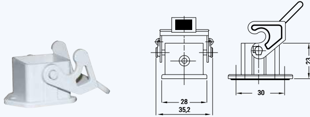
Montaj Eksenleri (22x22) Panel cut - out (22x22)
